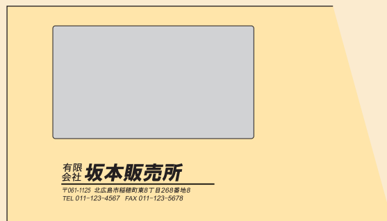
長形 4 号封筒&lt;窓付&gt; 寸法 90×205mm
